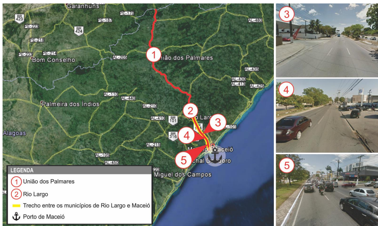
Figura 15. Pontos Críticos BR-104-AL
